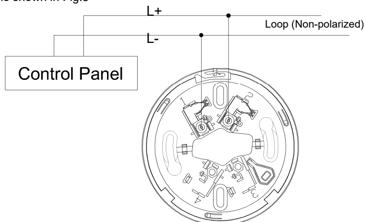
Fig.3. Loop wiring
